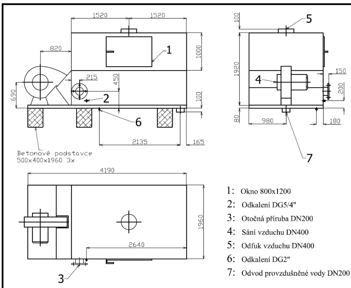
Obr. č2: Zástavbové rozměry BUBLA 25V
