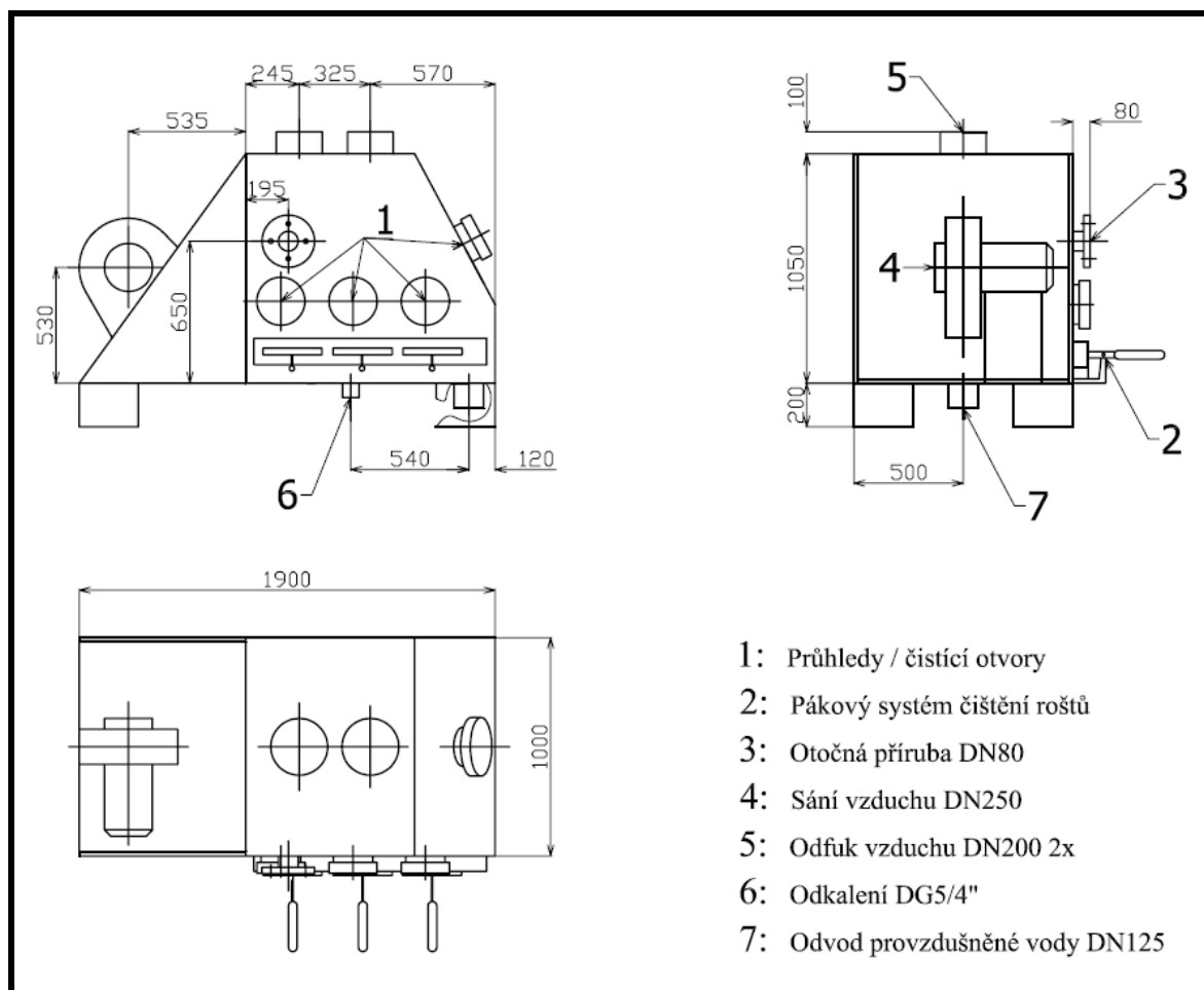
Obr. č2: Zástavbové rozměry BUBLA 5V
